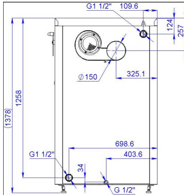
Фигура 5.3. Изглед към входно/изходните щуцери на котел "Pelletherm 45 V.2 M03".
