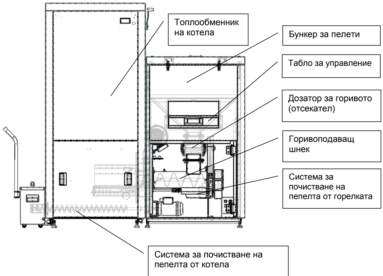
Figure 4.4. Частичен разрез на котел "Pelletherm 100 V.2 M03" – поглед отпред.
