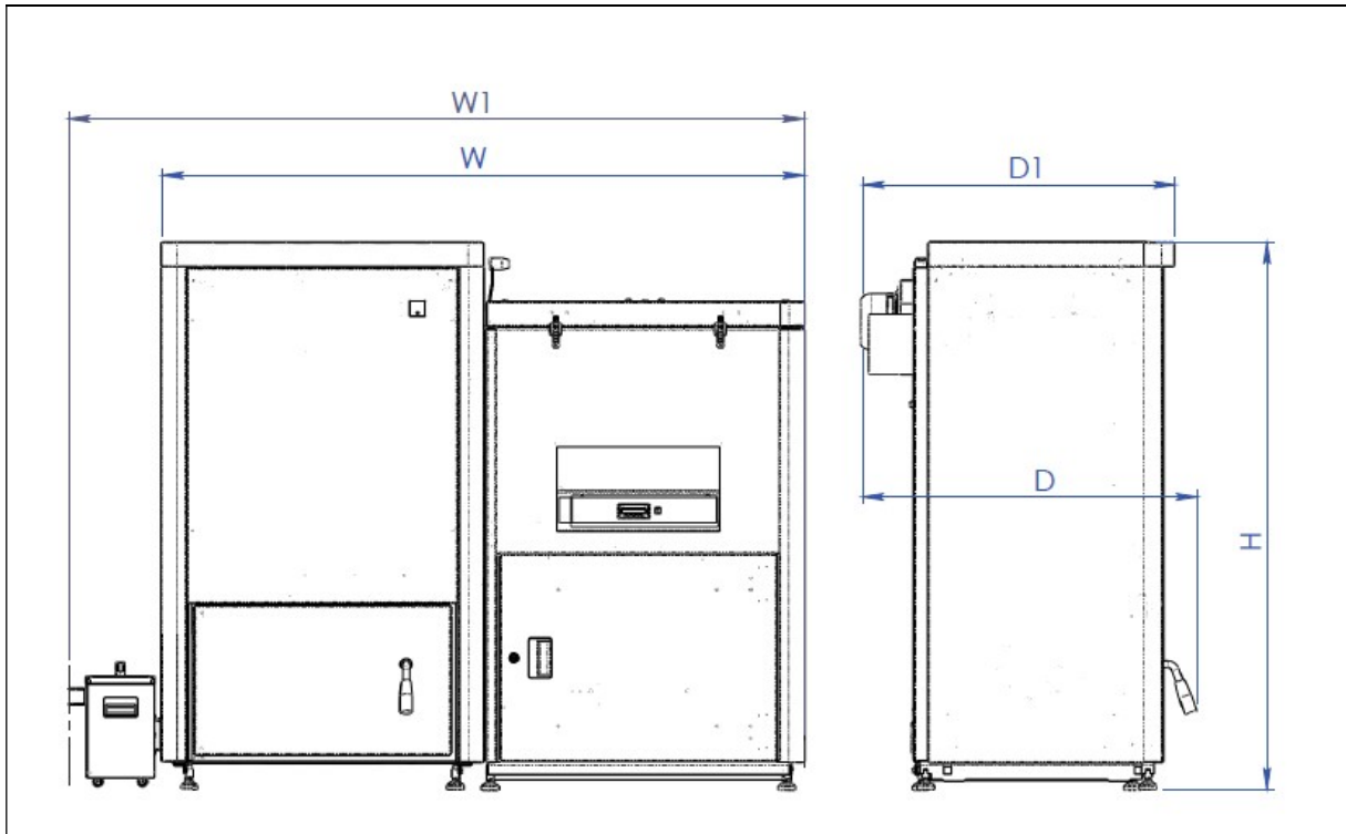
Фигура 3.1. Размери на котел серия "Pelletherm V.2 M03".
